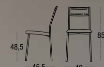
SILLA ALOHA 45 ASIENTO TAPIZADO TUBO CUADRADO METÁLICO DE 20
