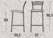
TABURETE MEDIO MARTA 65 ASIENTO TAPIZADO TUBO REDONDO METÁLICO Ø 25
