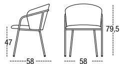
SILLÓN SEDA 4530 ASIENTO Y RESPALDO TAPIZADO TUBO REDONDO METÁLICO Ø18
