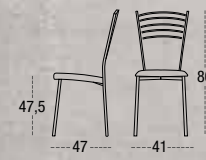
SILLA MARTA 45 ASIENTO TAPIZADO TUBO REDONDO METÁLICO Ø 25
