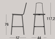
TABURETE ALTO BONN 7503 CARCASA TAPIZADA PATA REDONDA METÁLICA Ø18
