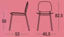
SILLA NIZA ASIENTO Y RESPALDO TAPIZADO CHASIS REDONDO METÁLICO Ø 22
